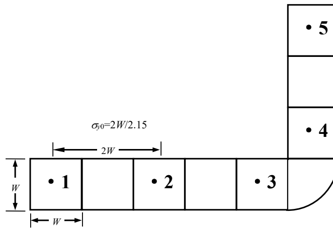
图 C. 4 连续划分的体源
